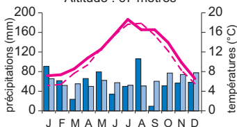
Station météorologique de Caen-Carpique (Calvados) Altitude : 67 mètres
